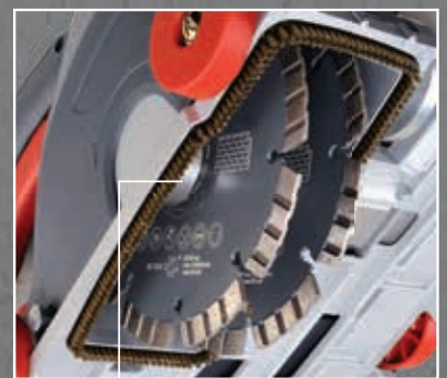
2 blades
